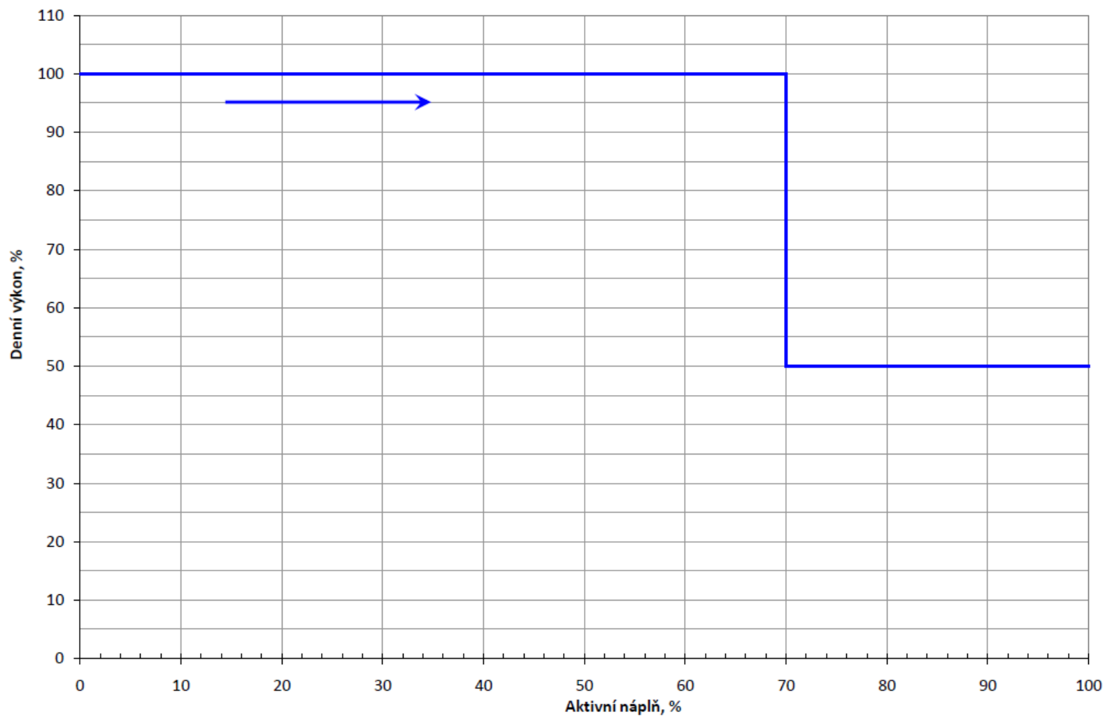
Vtláčecí výkonová křivka (10 mil. m 3 )
